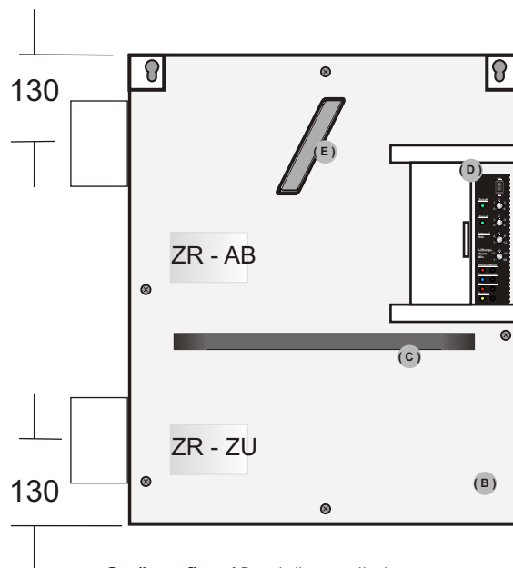
- Geräteaufbau (Darstellung mit abgenommener Dekorblende) :
