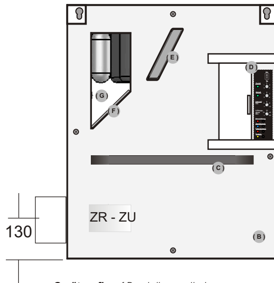
- Geräteaufbau ( Darstellung mit abgenommener Dekorblende ) :
