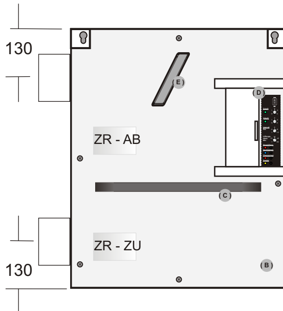
- Geräteaufbau (Darstellung mit abgenommener Dekorblende) :
