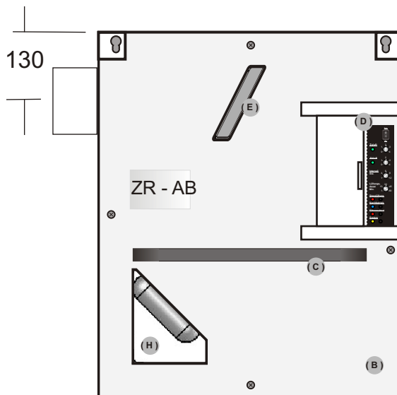
- Geräteaufbau (Darstellung mit abgenommener Dekorblende) :
